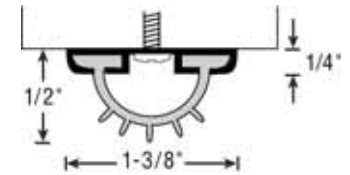
774S Door Edge Mill/Vinyl
