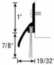
770SB Door Sweep w/Drip Cap Mill/Brush
